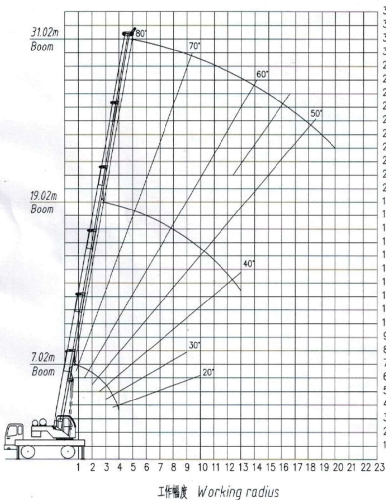
STSQ10A起升高度曲线 (LIFTING HEIGHT CURVE)
